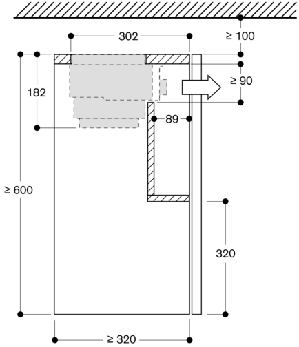
Querschnitt von Oberschrank für AF210 mit AA 211 812
