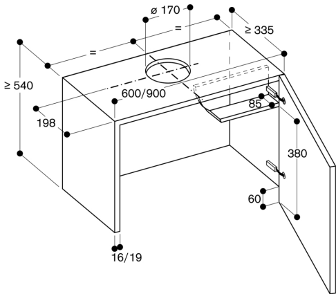
Oberschrank für AF 210 mit Absenkrahmen
