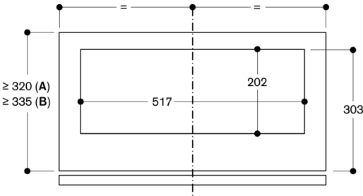
Ansicht von Oberschrank von oben mit AA 211 812
