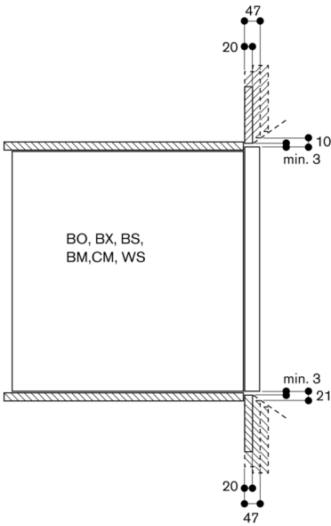
Luftquerschnitte an den Türkanten oben/unten
