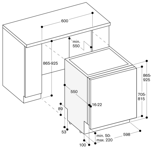
86,5 cm hoher Geschirrspüler mit flexiblem Scharnier
